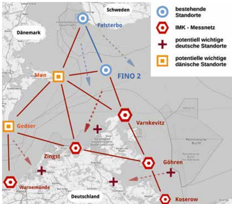
Abb. 1: Die Messanordnung für die stationäre Radiotelemetrie von Vögeln im Ostseeraum war bislang auf zwei Standorte beschränkt: Falsterbo/Schweden und Offshore-Plattform FINO 2 (siehe Sjöberg et al. 2015). Es ist vorgesehen, entlang der Küste Mecklenburg-Vorpommerns unter Nutzung der bestehenden Infrastruktur des Internen Messnetzes Küste (IMK) zusätzliche Empfangsstationen (Warnemünde, Zingst, Varnkevit, Göhren, Koserow) zu installieren. Diese Stationen würden in annähernd äquidistanter Anordnung zusammen mit den bisher installierten Stationen und weiteren Stationen in Dänemark (Gedser, Møn) ein untereinander kalibrierbares Messnetz bilden. Zusätzliche Standorte in Deutschland (rote Kreuze) sind aus ornithologischer Sicht von besonderem Interesse (blaue gestrichelte Vektoren: bisher dokumentierte Abflugrichtungen im Herbst; rote gestrichelte Vektoren: über Triangulation messbare, potenzielle Zugwege).
